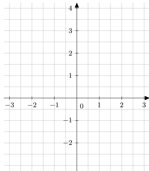
Das Schaubild der Ableitungsfunktion
