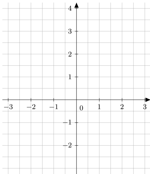
Das Schaubild der Ableitungsfunktion
