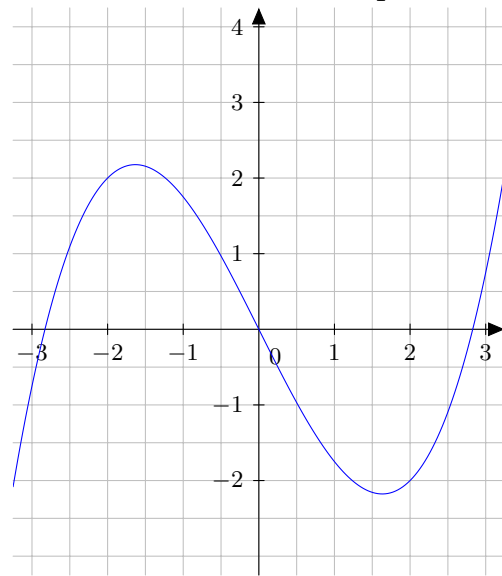
Das Schaubild von f(x) = \frac{1}{4}x^3 - 2x
