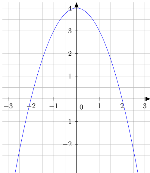
Das Schaubild von f(x) = 4 - x^2
